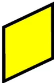
rhombus
